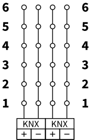
Схема подключения
