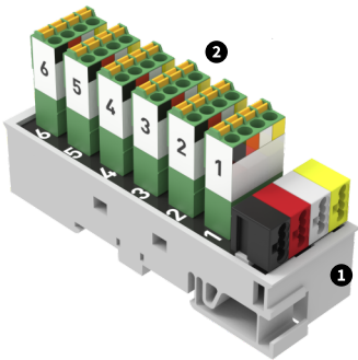
1. Клеммы шины KNX 2. Клеммы для кабелей ответвления
